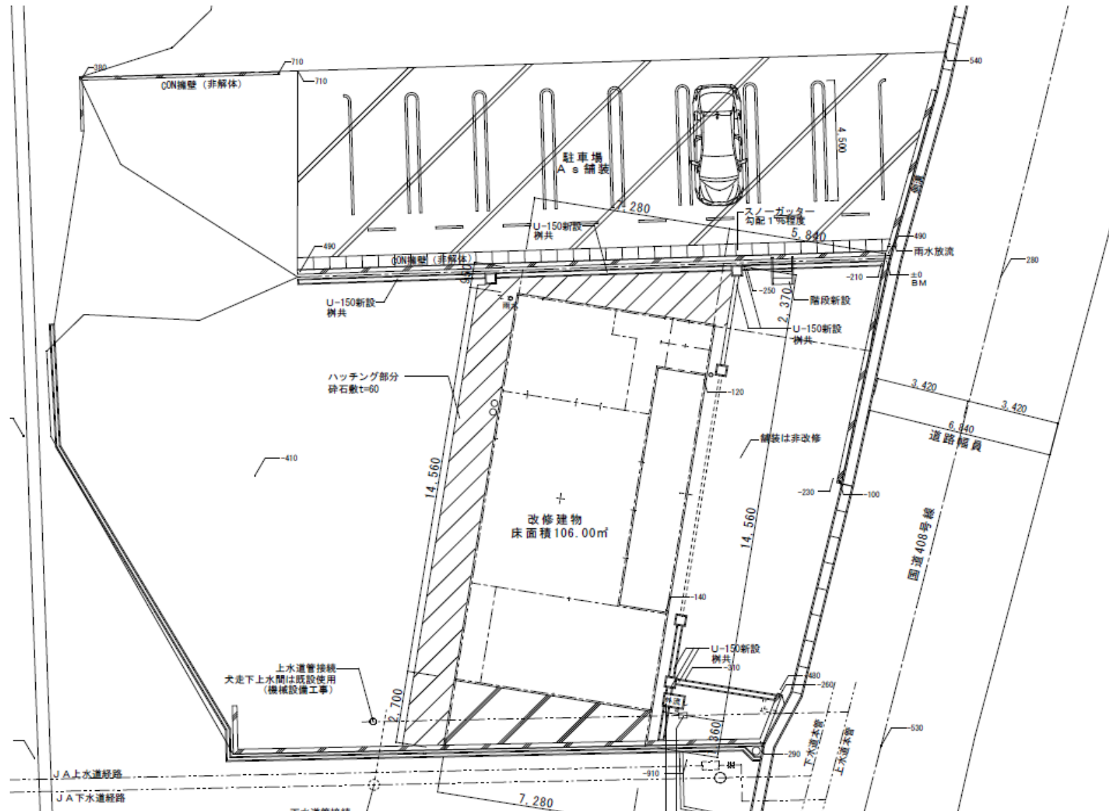
麻績村食堂交流施設外構図
