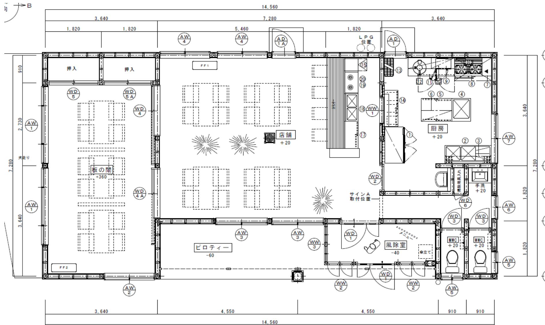
麻績村食堂交流施設平面図
